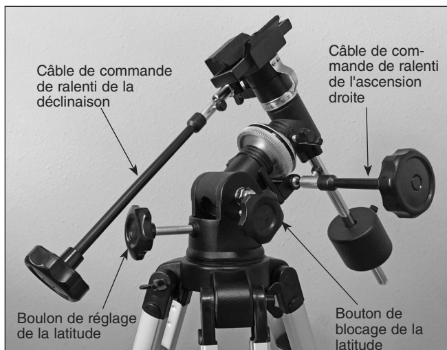
Figure 11. Vue arrière de la monture équatoriale, avec les deux câbles de commande de ralenti fixés.
