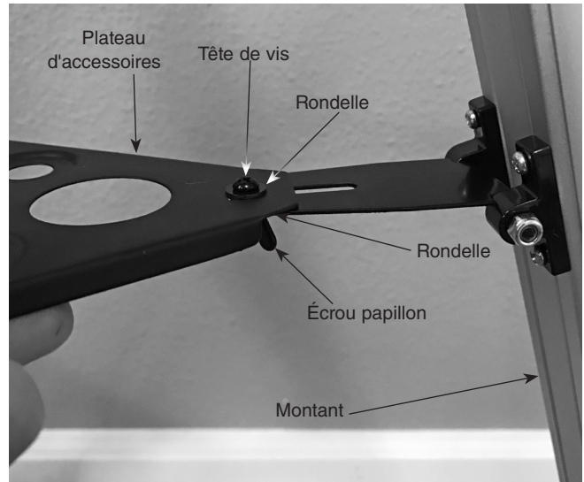
Figure 5. Attachez le plateau à accessoires à chacune des traverses de maintien des trois montants du trépied en utilisant le matériel fourni.
