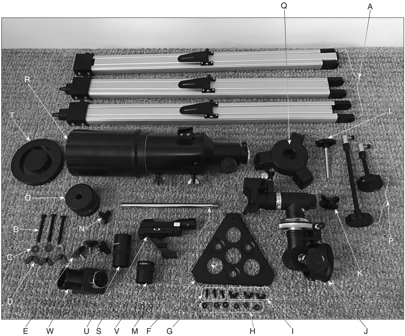
Figure 1. Les pièces du télescope équatorial Observer 80ST.
