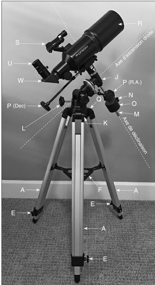
Figure 2. Le télescope équatorial Observer 80ST entièrement assemblé, avec les pièces clés identifiées.
