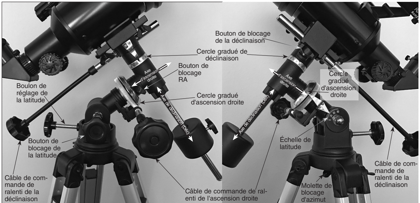
Figure 18. Composants de la monture équatoriale, vus des deux côtés.
