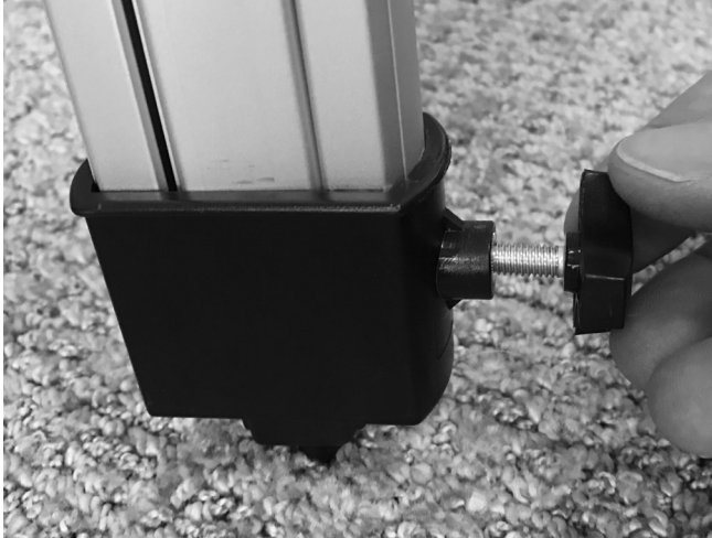
Figure 4. Enfilez une vis de verrouillage de montant sur chaque montant du trépied comme indiqué, en veillant à ne pas trop serrer.
