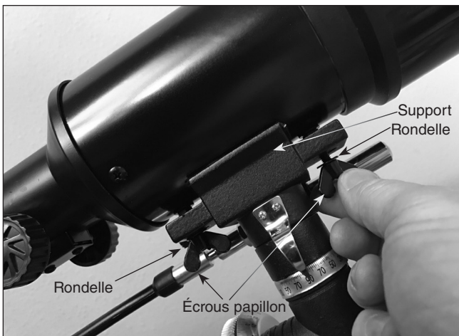
Figure 14. Fixez le tube optique à la plaque de support de la monture avec les écrous papillon et les rondelles fournis.
